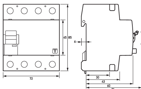
Maßzeichnung Fehlerstromschutzschalter DFS 4 063-4/0,30-HP
