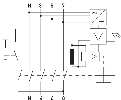
Schaltungsbeispiel Fehlerstromschutzschalter DFS 4 063-4/0,30-HP
