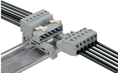
Federleiste; mit Rastfüßen und Montageadapter 209-137; auf Tragschiene 35
