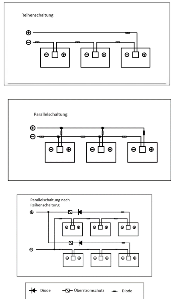
Abb. 13 Schaltbild der elektrischen Anschlüsse
