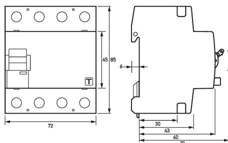
Maßzeichnung Fehlerstromschutzschalter DFS 4 063-4/0,30-PV
